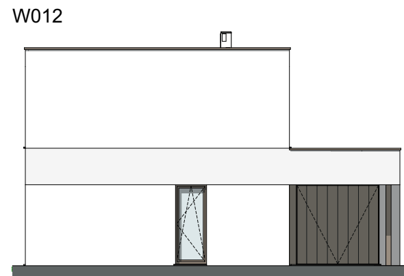
Linkergevel 1:150
