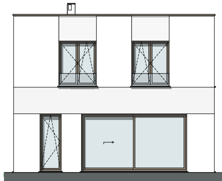
Achtergevel 1:150
