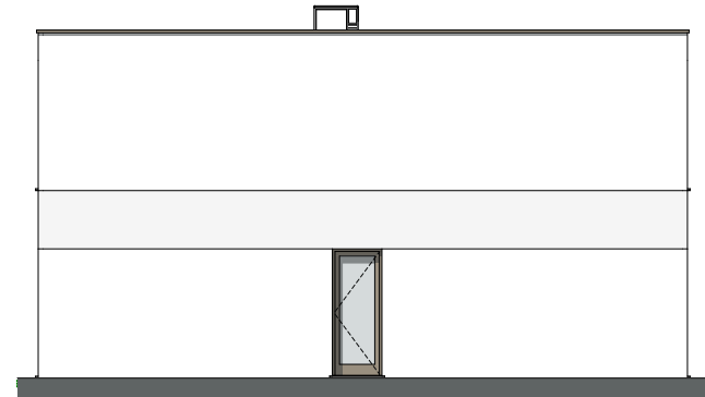
Rechtergevel 1:150
