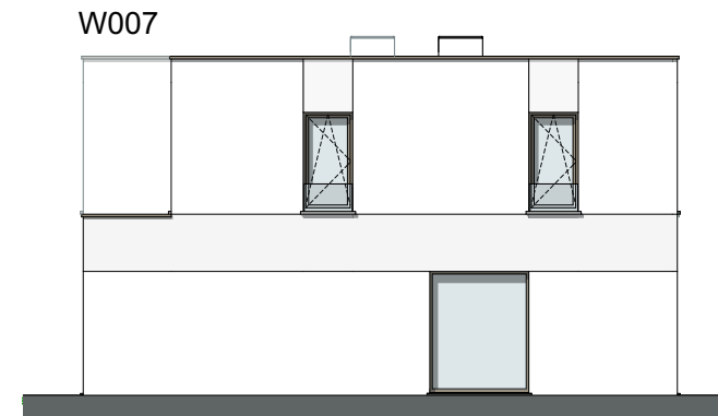
Linkergevel 1:150
