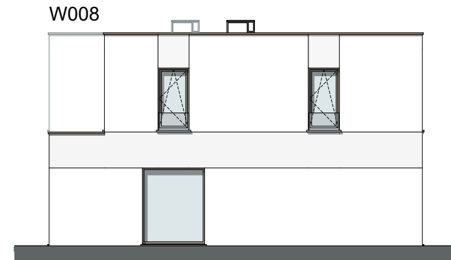
Rechtergevel 1:150
