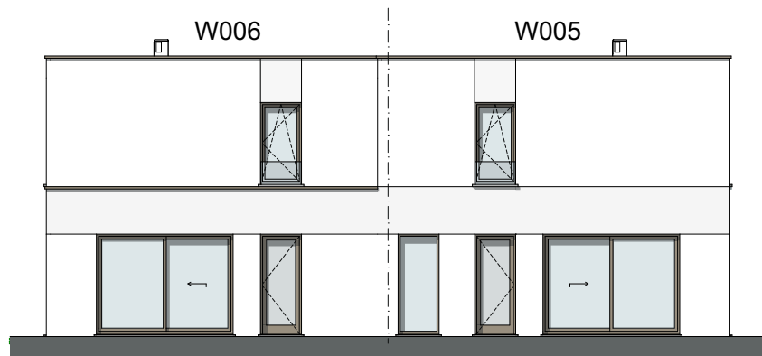
Achtergevel 1:150
