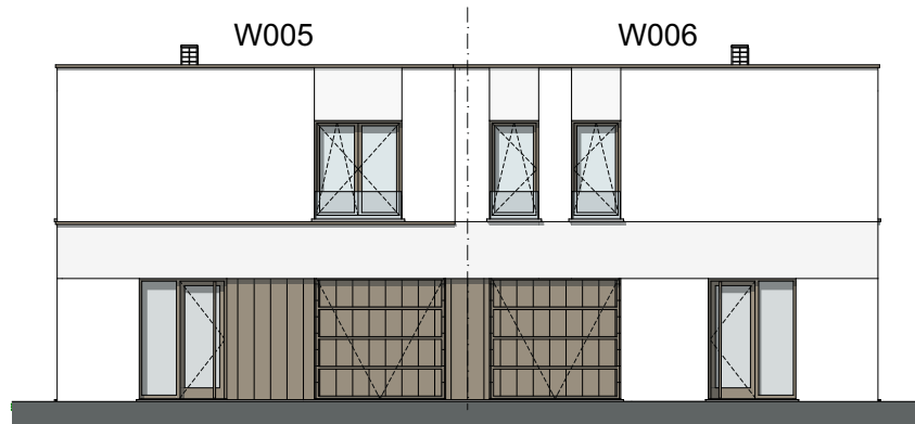
Voorgevel 1:150
