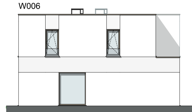
Rechtergevel 1:150
