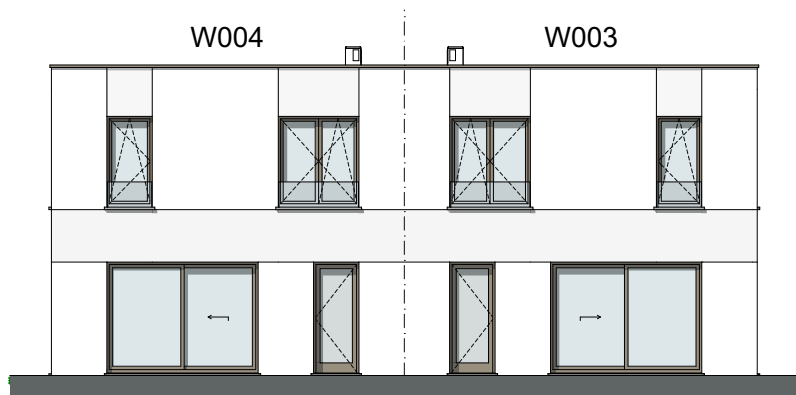
Achtergevel 1:150
