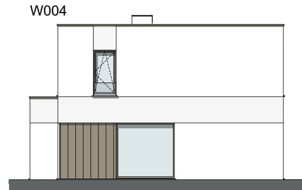
Rechtergevel 1:150
