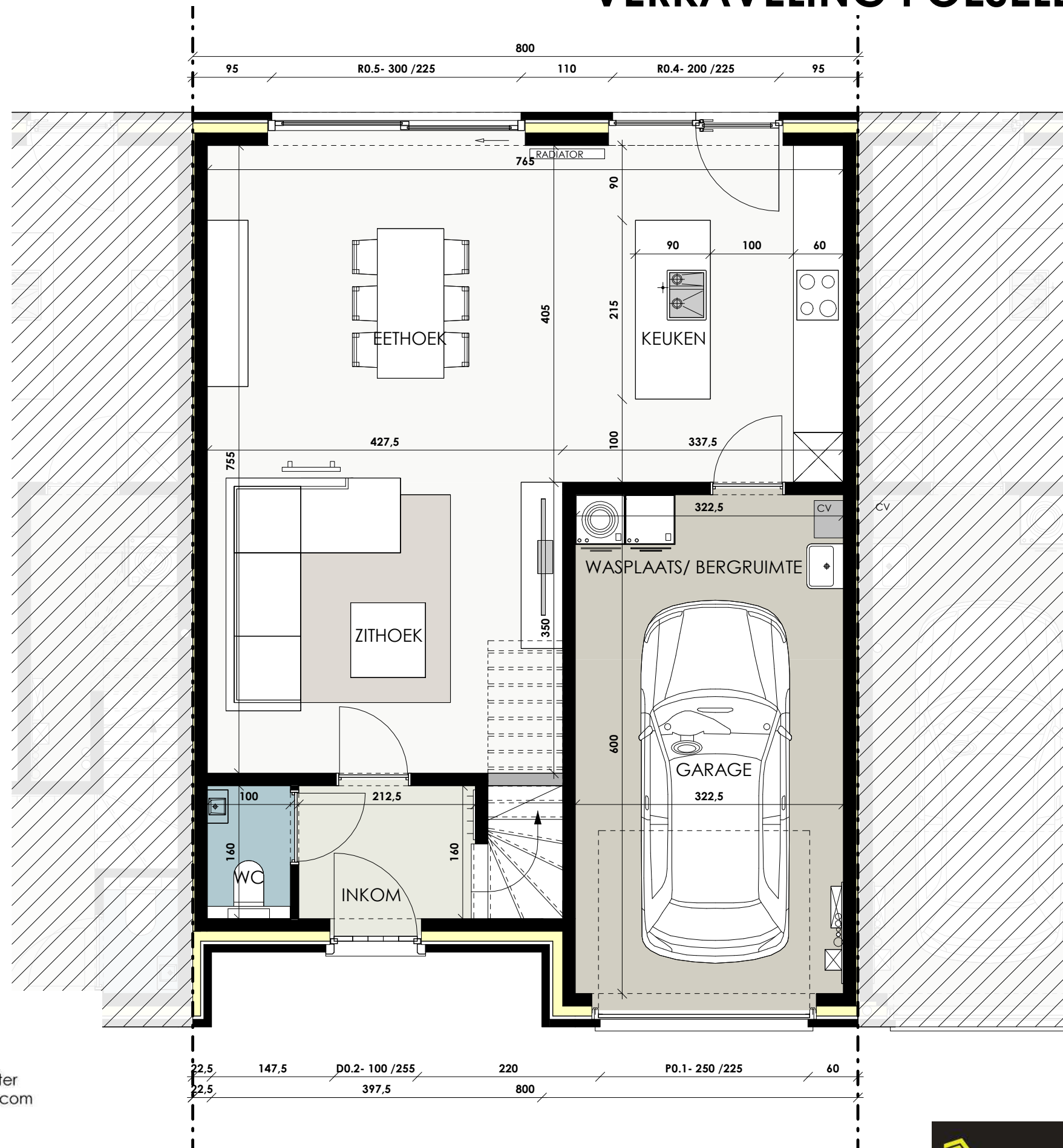
GRONDPLAN LOT 32
