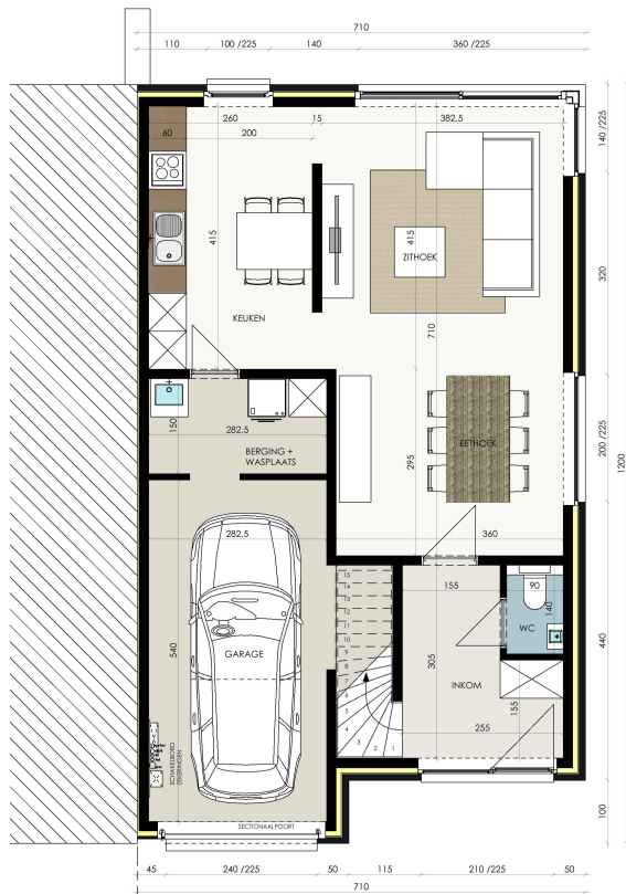
GRONDPLAN LOT 3
