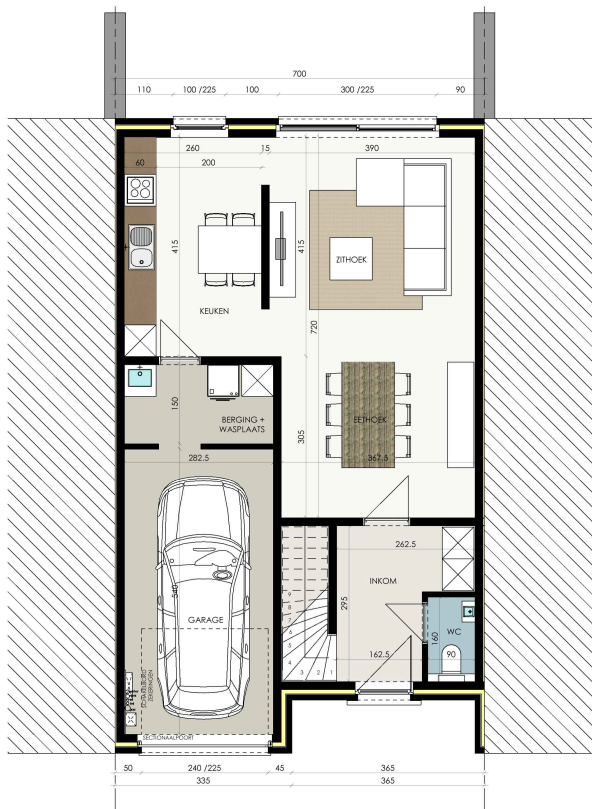
GRONDPLAN LOT 16
