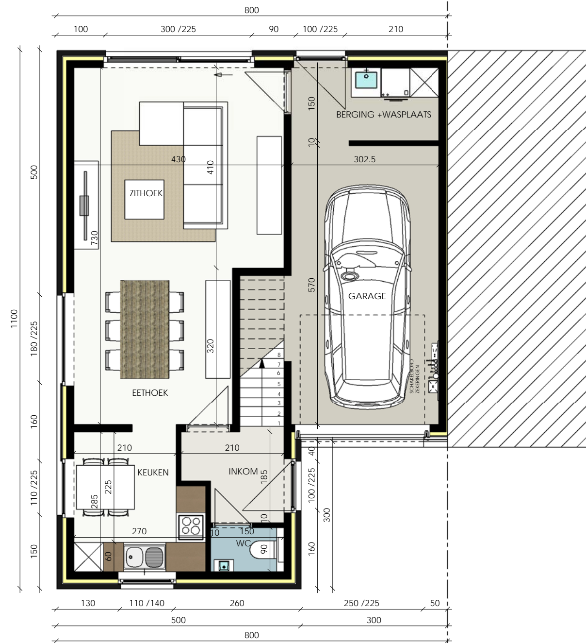
GRONDPLAN LOT 4
