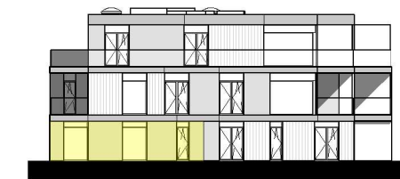
Gevel zuidwest
